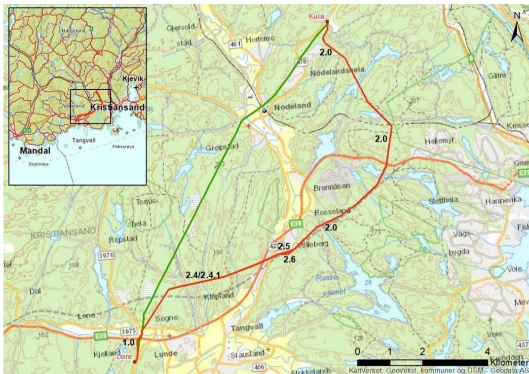
Figur 4-8: Konsesjonssøkt ny ledning er vist med rød linje. Grønn linje er dagens Kulia - Leire som er omsøkt revet. Kilde: Glitre Nett.
