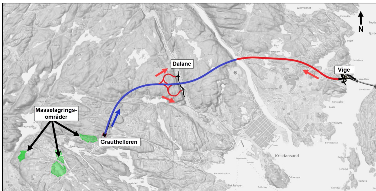
Figur 6-21: Drivekonsept for Ytre ringvei. Blå linjer viser rigg med utgangspunkt fra Grauthelleren. Rød linje viser rigg med utgangspunkt fra Vigje, som senere flyttes for å drive rampe- og tilførselstunneler ut til Dalane.
