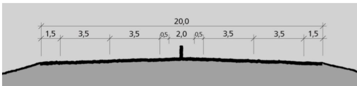
Figur 6-2: Normalprofil for 4-felts motorvei i Vige.
