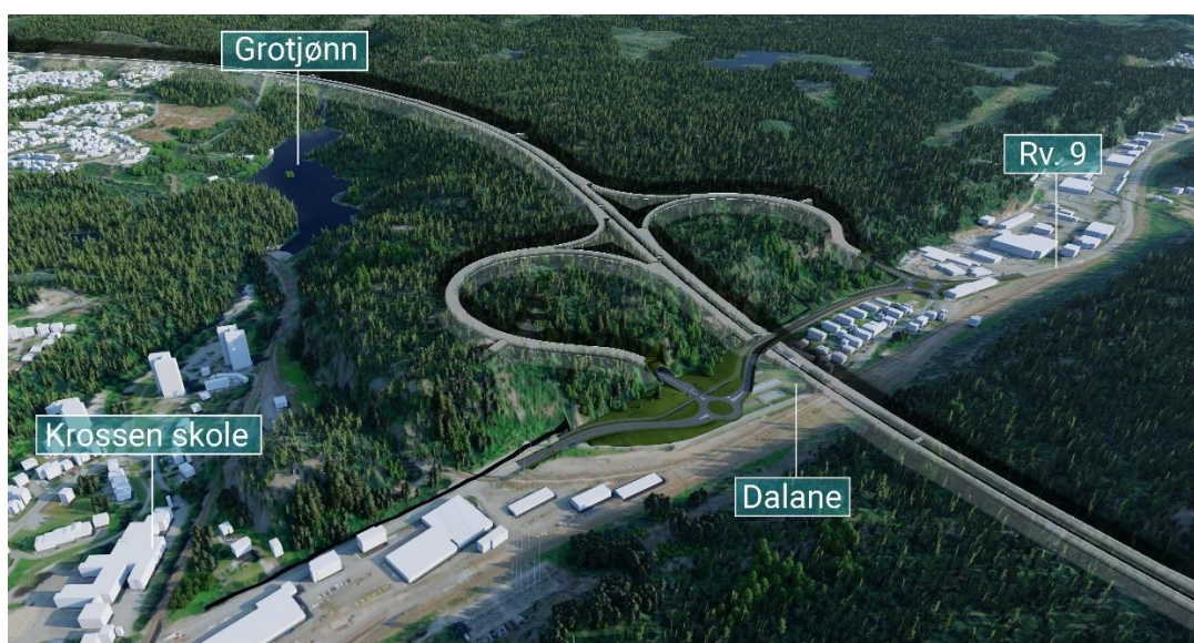
Figur 6-9: Kryss i tunnel, ved Dalane.
